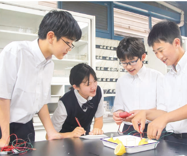
レモン電池実験(探究理科)
